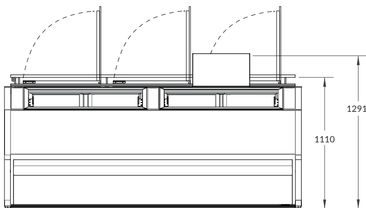
Vista superior
