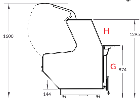
Vista Lateral
